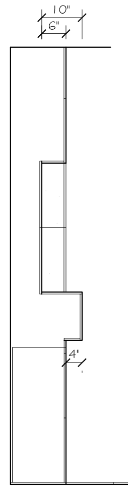
3 Section AA Scale: 1/2" = 1'-0"
