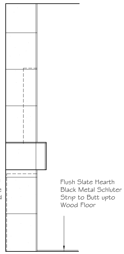
4 Side Elevation Scale: 1/2" = 1'-0"
