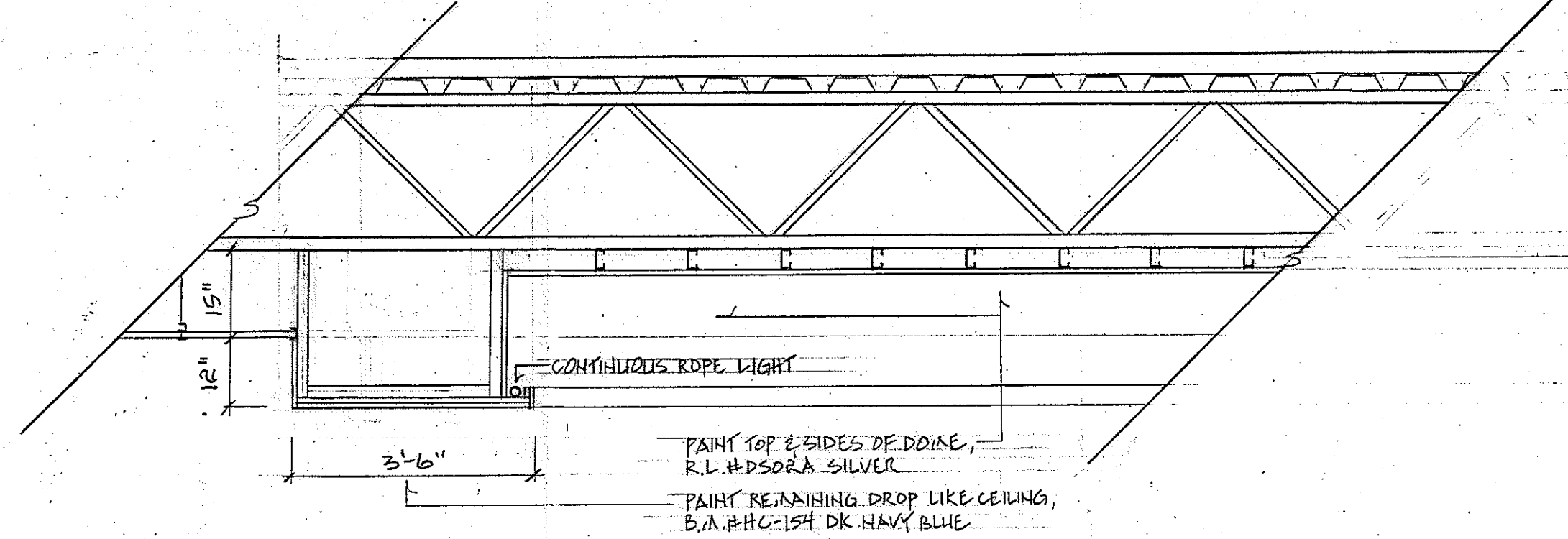
DOME SECTION ELEVATION SCALE: 1/2" = 1'-0"
